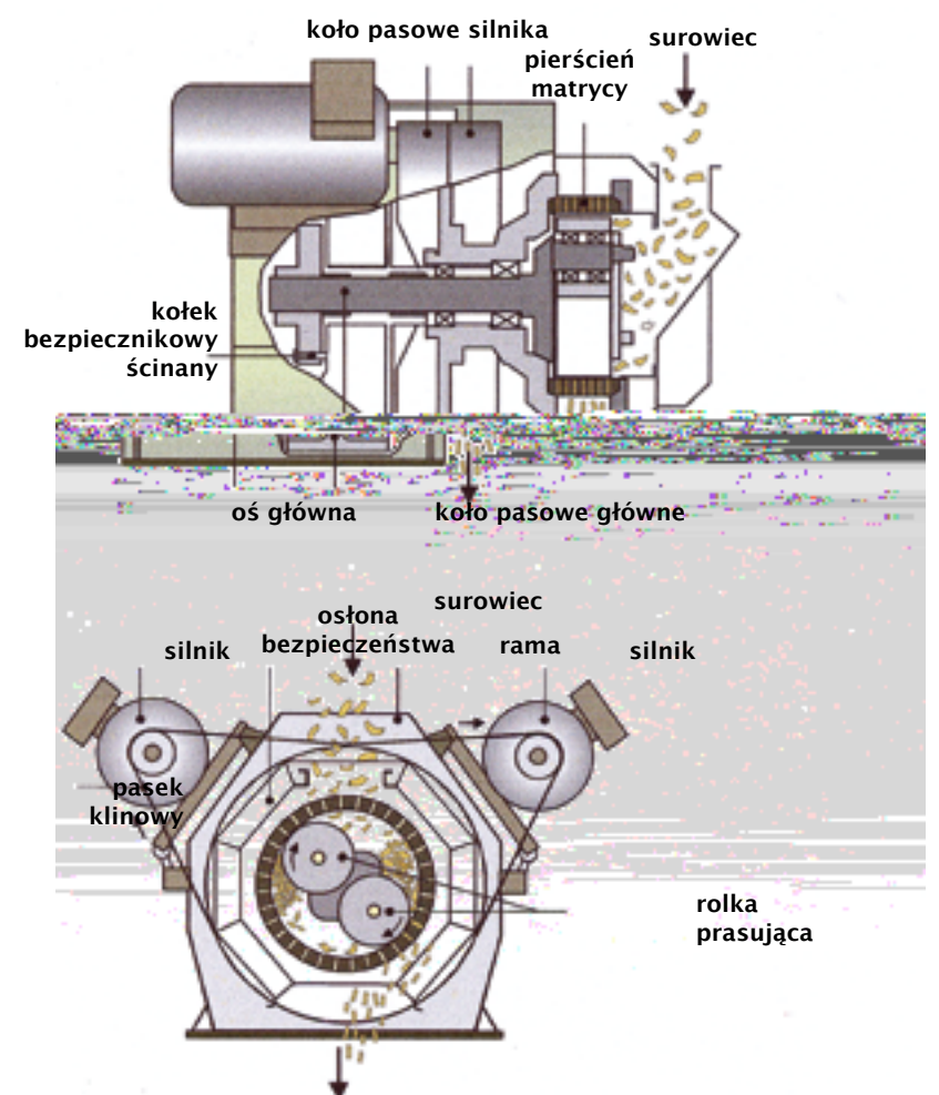
Rys. Pionowo mocowana matryca (źródło www.salmatec-gmbh.de)
